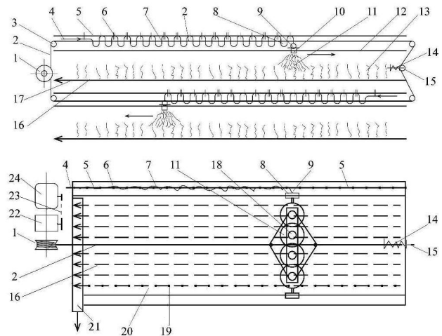
Նկ. 2. Կանաչ կերի արտադրության տեղակայանքի խոնավացման համակարգի կառուցվածքային սխեման (կազմվել է հեղինակների կողմից). 1 - բազմափայտության թվբուկ, 2 - մետաղաձուլակ, 3 - ուղղապատի հողովակներ, 4 - լուծույթի մատուցման խողովակ, 5 - մետաղական լար, 6 - մետաղական օղակներ, 7 - լուծույթի փողրակ, 8 - ցնցողատար անիվներ, 9 - անուր, 10 - ցնցողներ, 11 - կոնական շիթեր, 12 - կրող լար, 13 - աճեցվող բույս, 14 - զսպանակ, 15 - ձգող հողովակ, 16 - հարկաշարեր, 17 - ավելորդ լուծույթ, 18 - աշխատանքային օրգան, 19 - շաղափված անցքեր, 20 - առվակներ, 21 - կուտակիչ առվակ, 22 - ռետուկտոր, 23 - փոկային փոխանցում, 24 - էլեկտրաշարժիչ:
